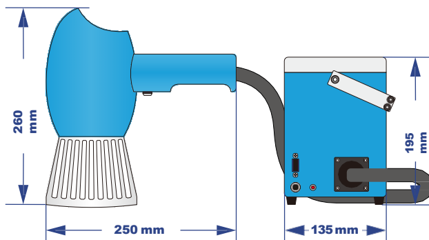
نمای جانبی
