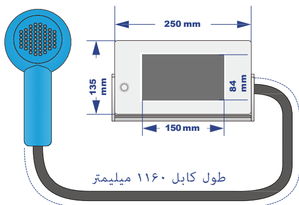
نمای بالا
