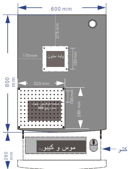
نمای بالایی
