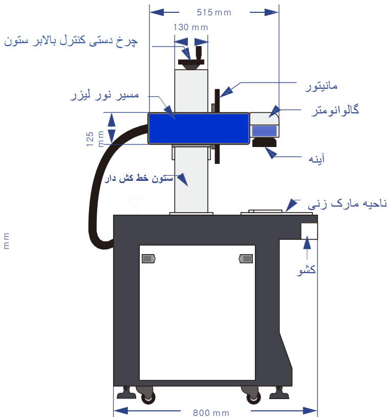
نمای کناری
