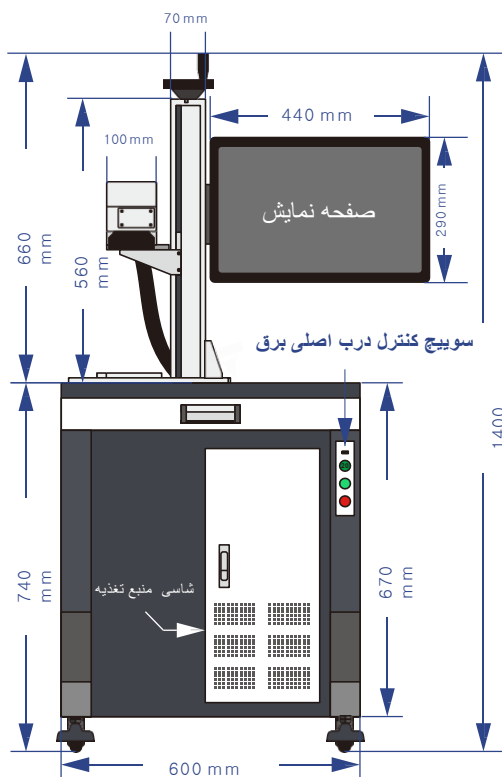
نمای جلویی
